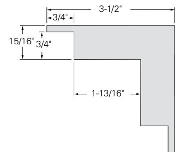
KLEER KONCEAL® CORNER
